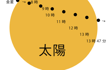
6月6日の金星太陽面通過の予測図
